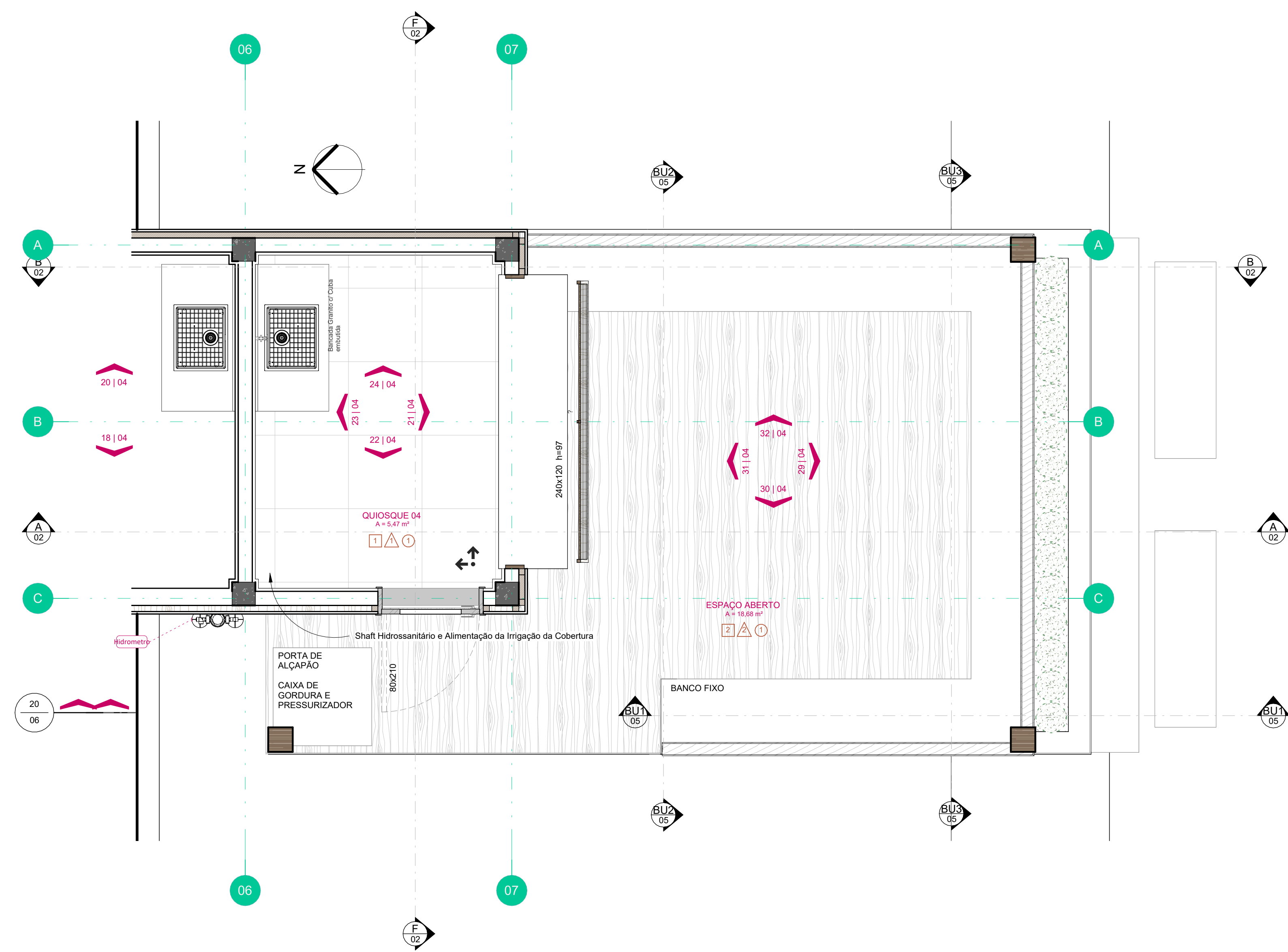
4 Quiosque 02 - Sem Cotas ESCALA: 1:25
