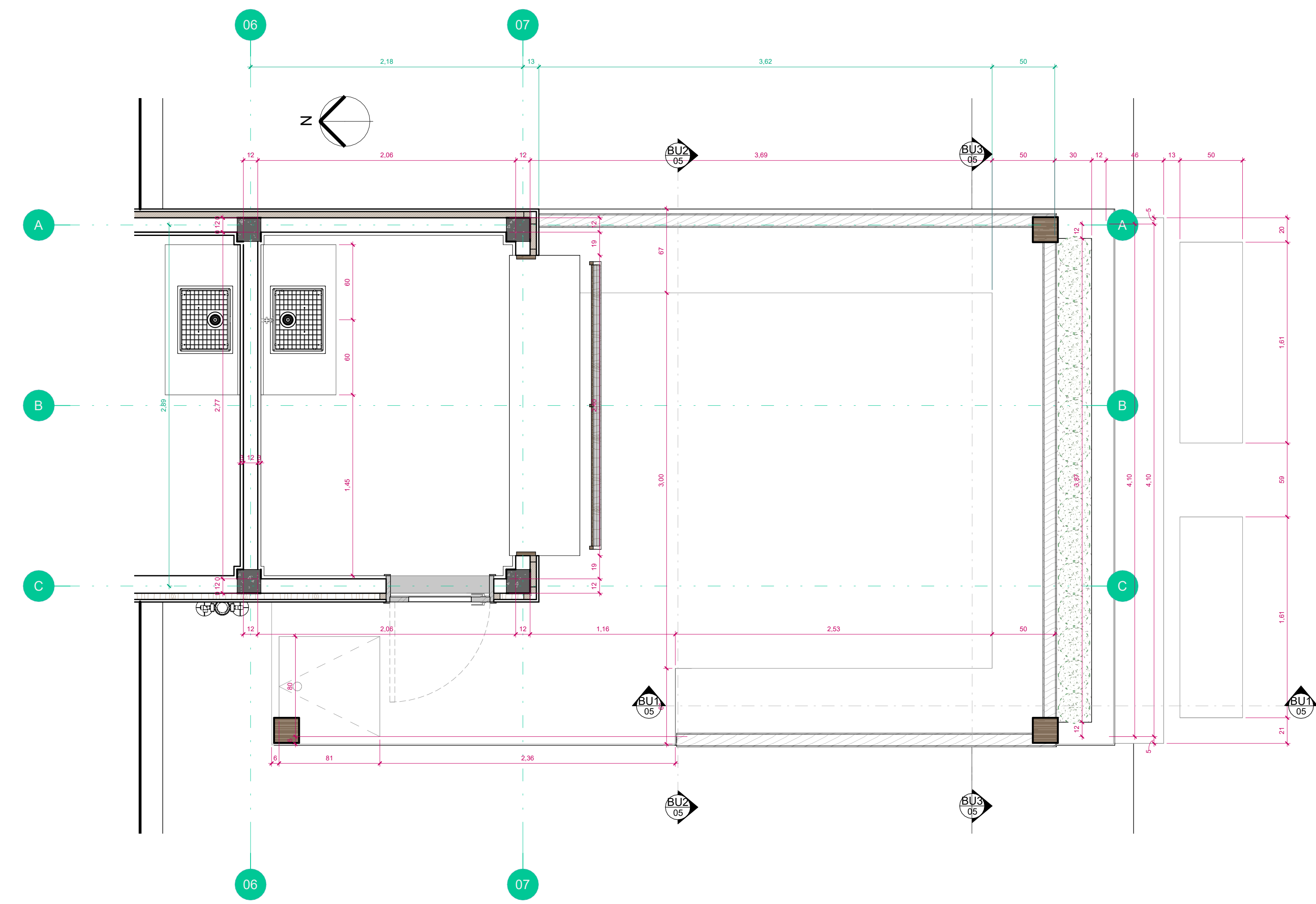
3 Quiosque 02 - Cotados ESCALA: 1:25
